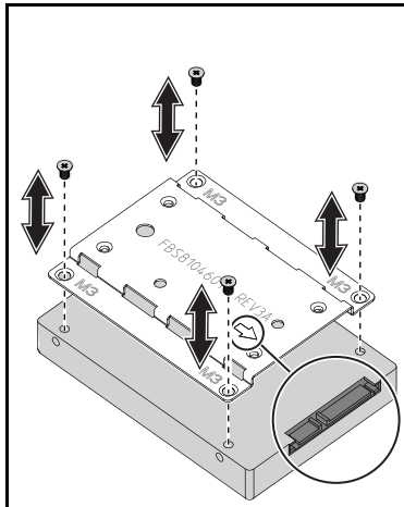
Ilustración 3-8. Extracción e instalación del soporte del disco duro de 2.5"
