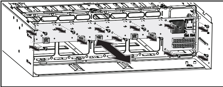
Ilustración 3-26. Extracción e instalación del plano posterior
